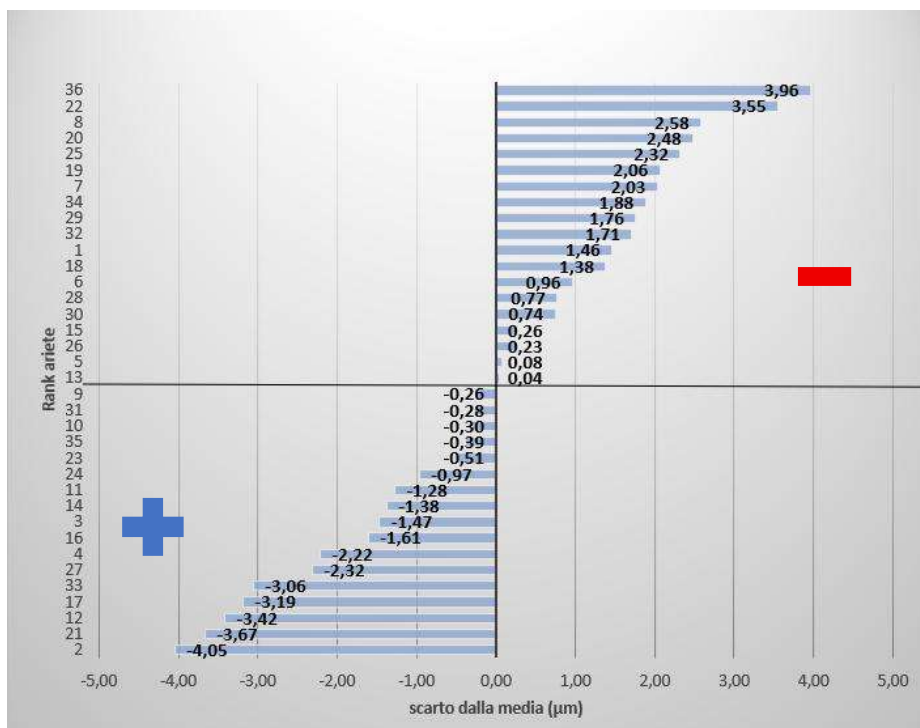
Grafico n. 1: Deviazione del diametro medio di ciascun individuo dalla media del campione analizzato
